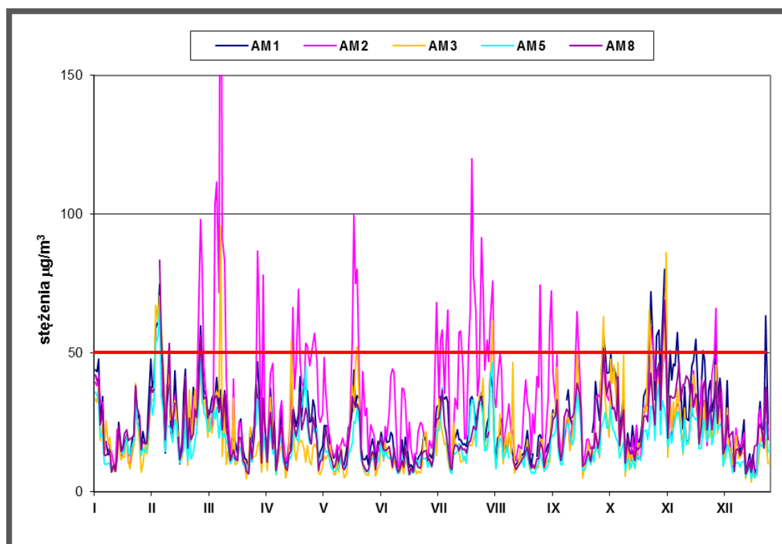
Ryc.50. Uśrednione średniodobowe przebiegi stężeń pyłu PM_{10} w roku 2014 w Gdańsku [ \mu g/m^3 ]
